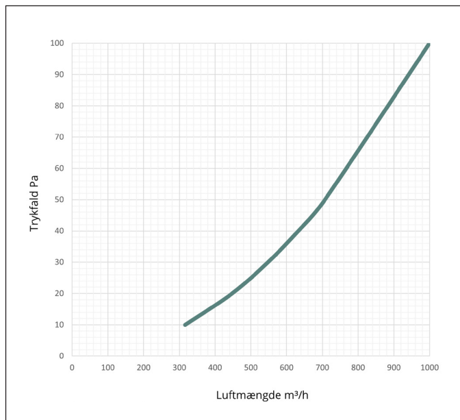
Kapacitetskurve Model A, K-faktor 100
