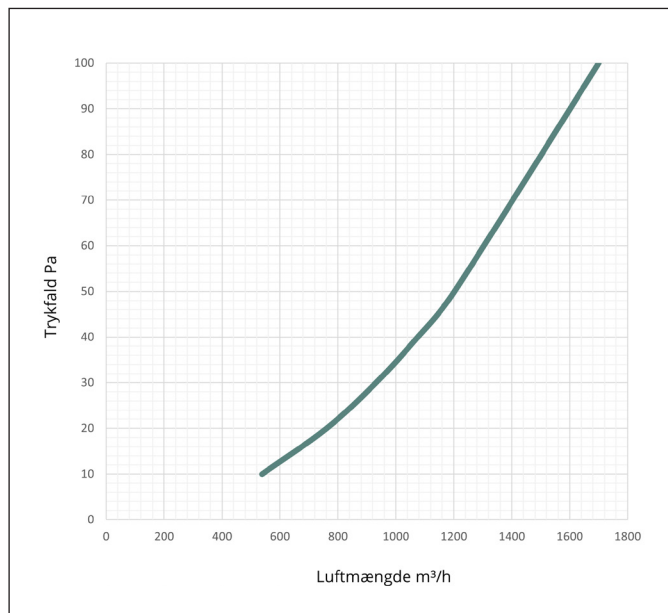
Kapacitetskurve Model B, K-faktor 170
